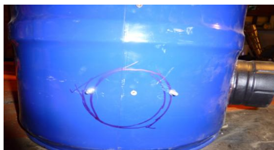
Tracé de l'ouverture maximum autorisée par la réservation : au centre la vis qui maintient le coffrage, de part et d'autre les 2 boulons déjà en place avant le coulage pour fixer la trappe.
