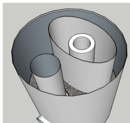
Éléments amovibles en métal : alimentation et redescende des fumées (cloche)
